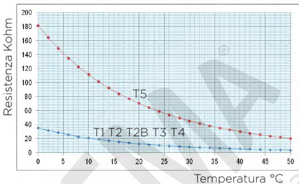
Tavola Temperatura/Resistenza Termistori (Sensori Temperatura)
