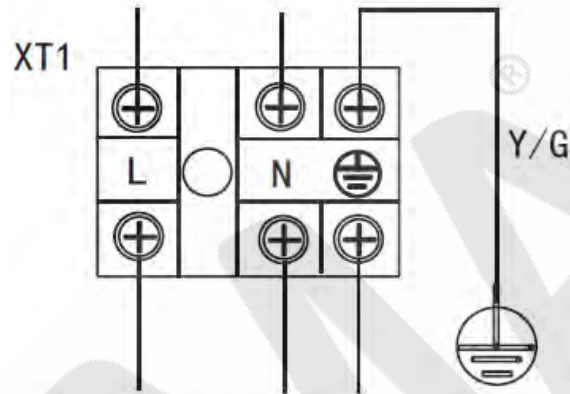
Alimentazione unità interna 220-240V / 1ph / 50Hz
