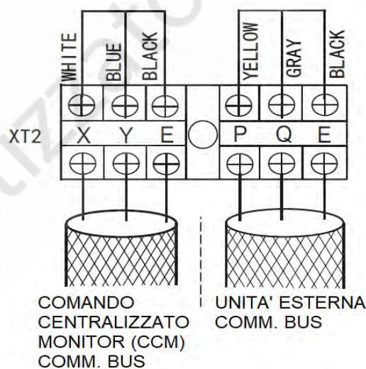
Utilizzare un cavo schermato a 3 conduttori
