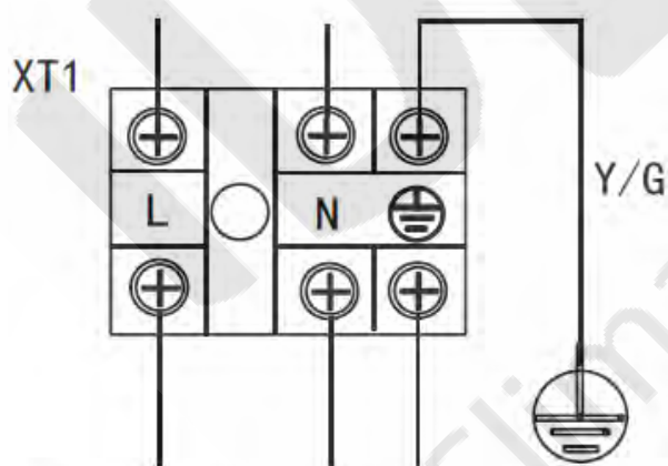
Alimentazione unità interna 220-240V / 1ph / 50Hz
