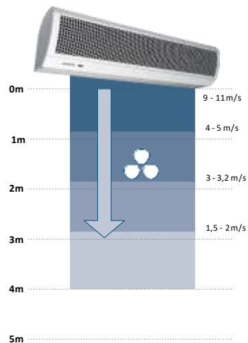
RENDIMENTO (VELOCITÀ DELL'ARIA) SERIE AC*-****SA1
